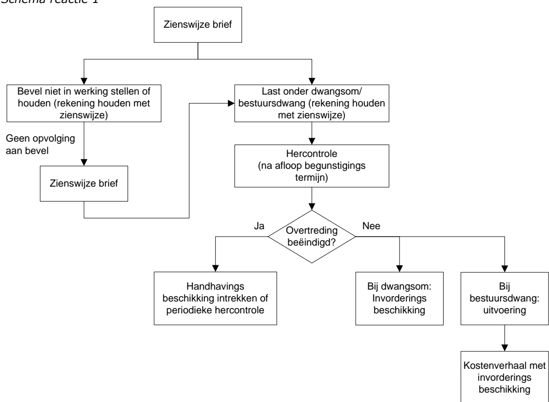
Schema reactie 1
