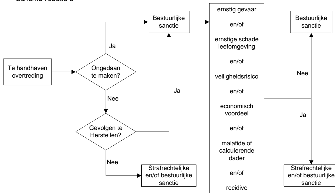
Schema reactie 3
